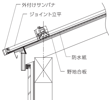
軒先納め
