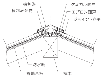
棟納め
