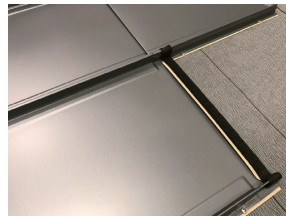
3 次列下段屋根 立上がり嵌合
