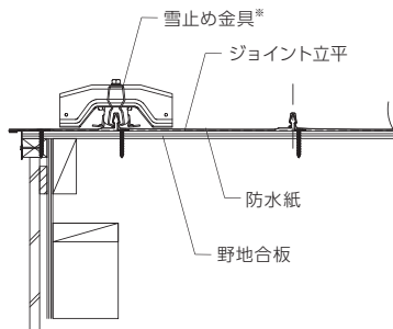
けらば納め
